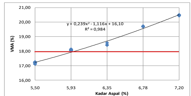
Gambar 9. Grafik Hubungan VMA dan Kadar Aspal Lataston HRS- Base Gradasi Semi Senjang
