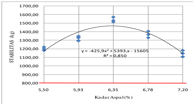
Gambar 5. Grafik Hubungan Stabilitas dan Kadar Aspal Lataston HRS-Base Gradasi Semi Senjang
