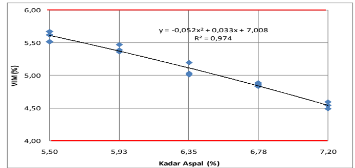
Gambar 3. Grafik Hubungan VIM dan Kadar Aspal Lataston HRS-Base Gradasi Semi Senjang
