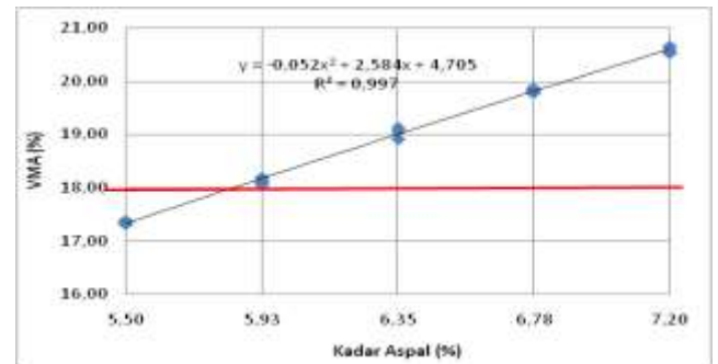
Gambar 8. Grafik Hubungan VMA dan Kadar Aspal Lataston HRS-Base Gradasi Senjang
